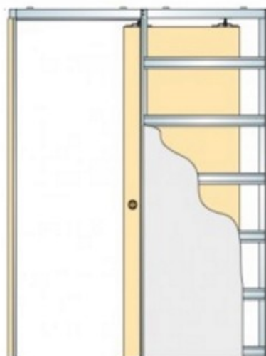
CONTROTELAIO ANTA UNICA A SCOMPARSA PER CARTONGESSO MOD. UNICO
