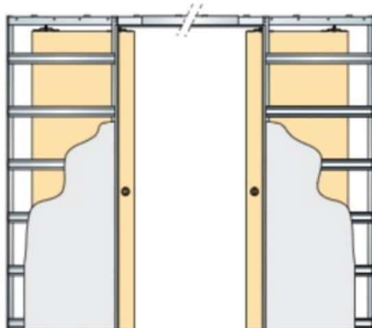
CONTROTELAIO ANTA DOPPIA A SCOMPARSA PER CARTONGESSO MOD. ESTENSIONE
